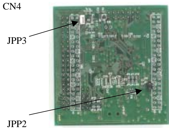
ハンダ面側
