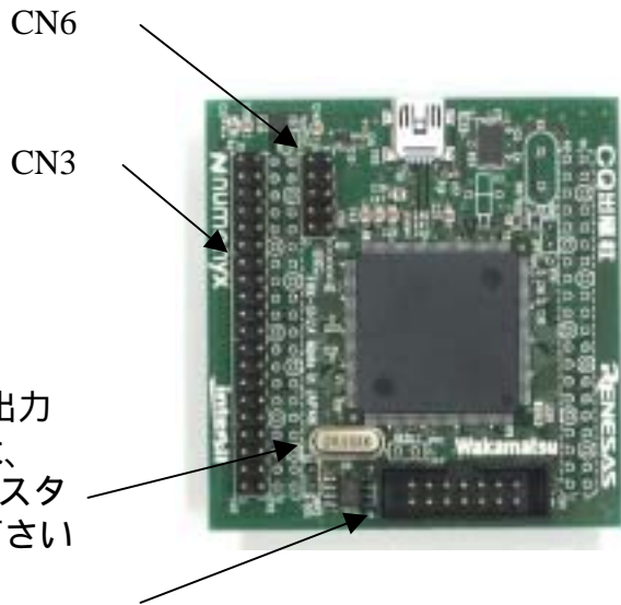
部品面側
